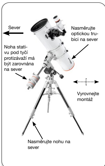
Obr. 16 a: Základní polární poloha, boční pohled.
