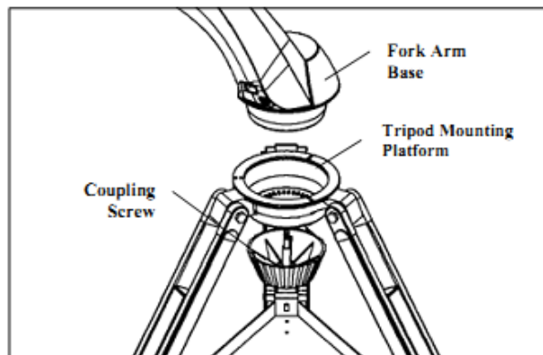
Obrázek 2.4 – montáž základny teleskopu
