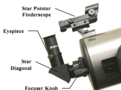
Obrázek 2.6 – Připojení okuláru (modely 90 a 127MAK)
