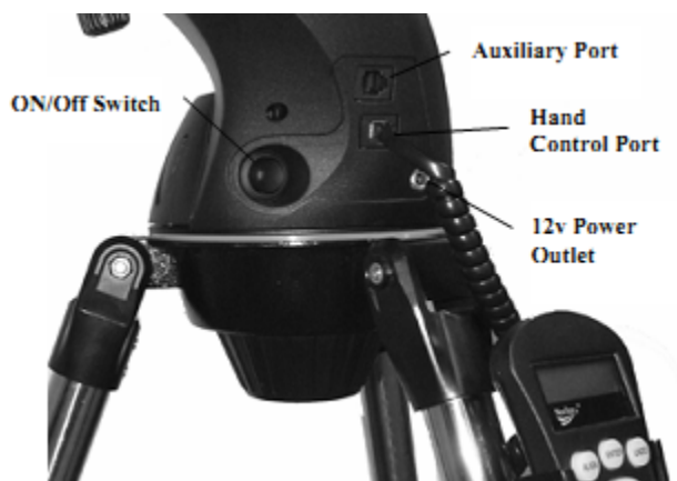
Obrázek 2.10 – Motorizovaná základna
