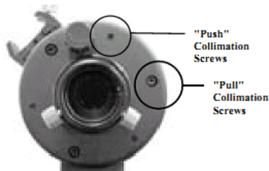
obr. 6.4 Ovládání kolimace: tlačítka („push“) kolimace, táhla („pull“) kolimace
