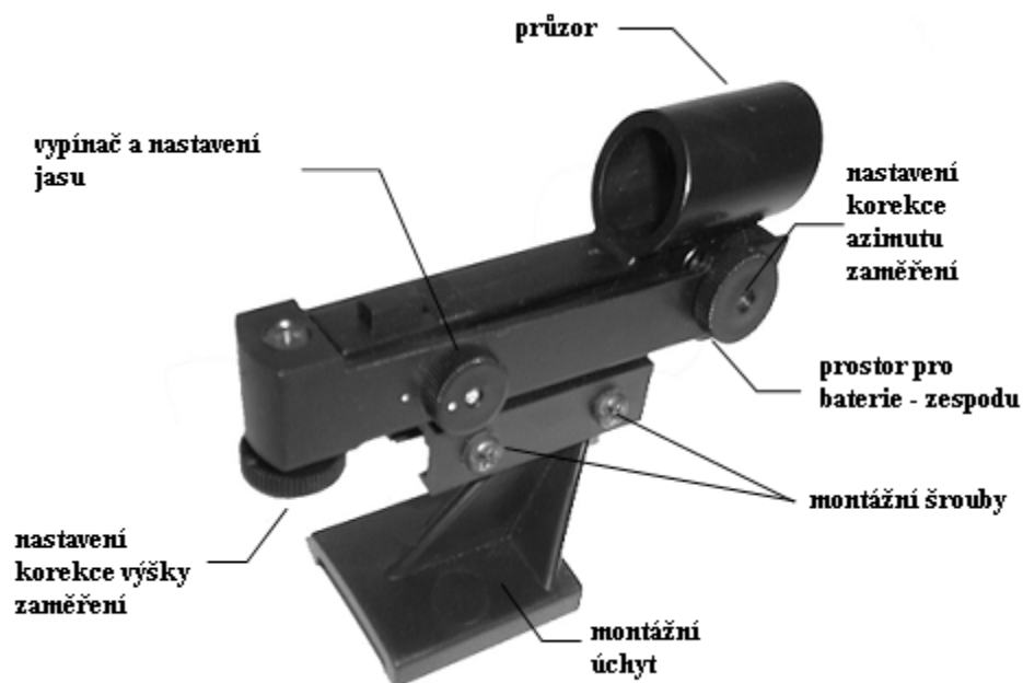
Obrázek 2.7 – Popis hledáčku StarPointer
